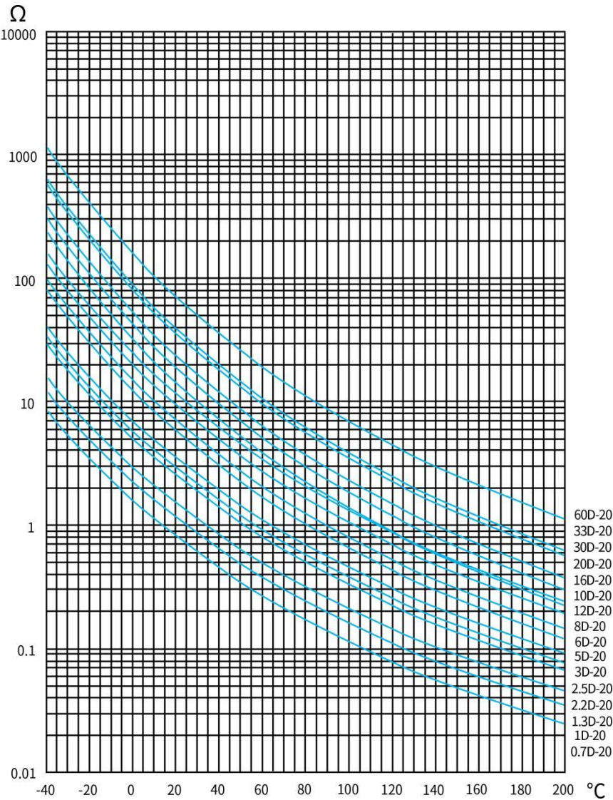
静态伏安特性曲线 Static Characteristics
