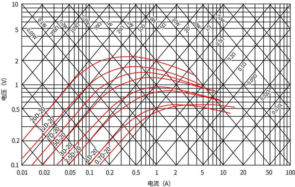
XXD-20电压-电流曲线
